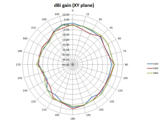
5GHz H-Plane
