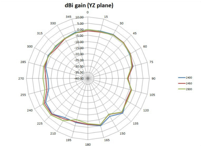
2.4GHz E-Plane
