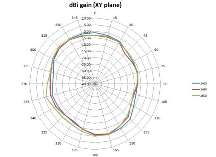
2.4GHz H-Plane
