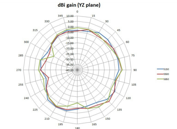
5GHz E-Plane
